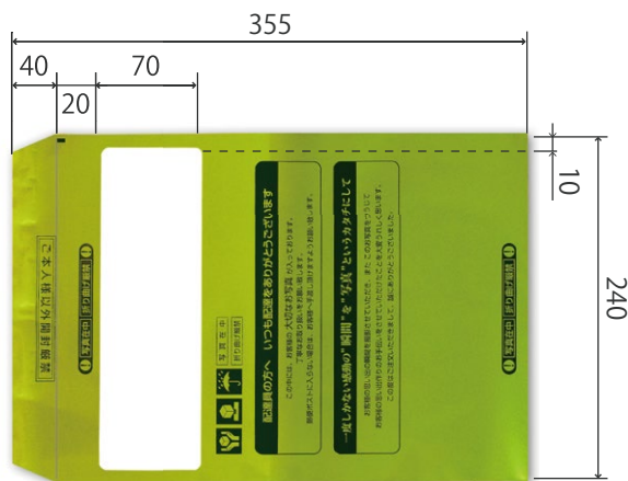
図. 楽しく梱包材 (大) ※ 6PW まで対応
